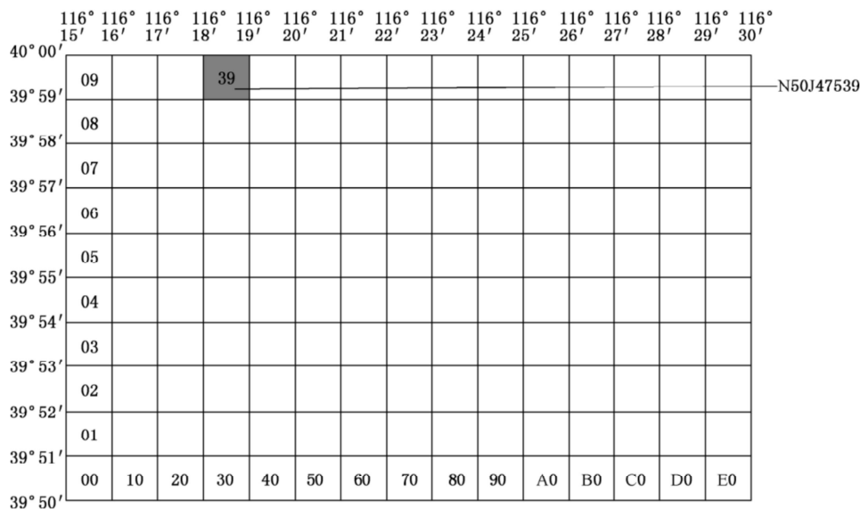
图 B.4 第四级北斗二维网格位置码
