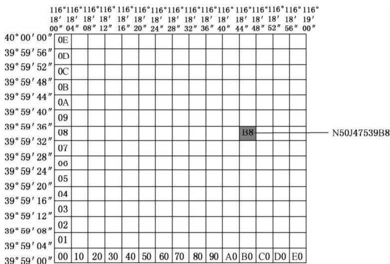
图 B.5 第五级北斗二维网格位置码
